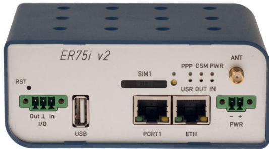
Basis Version im Kunststoffgehäuse mit 1 SIM-Karte und 1 Erweiterungsport
